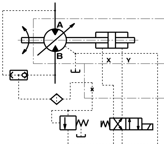
Внутреннее управление Питание клапана двух рабочих объемов от давления мотора
