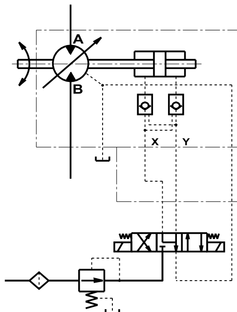
Внешнее управление Электромагнитный клапан регулирования рабочего объема с питанием от давления мотора
